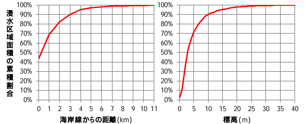
今回の津波浸水区域の地形条件
