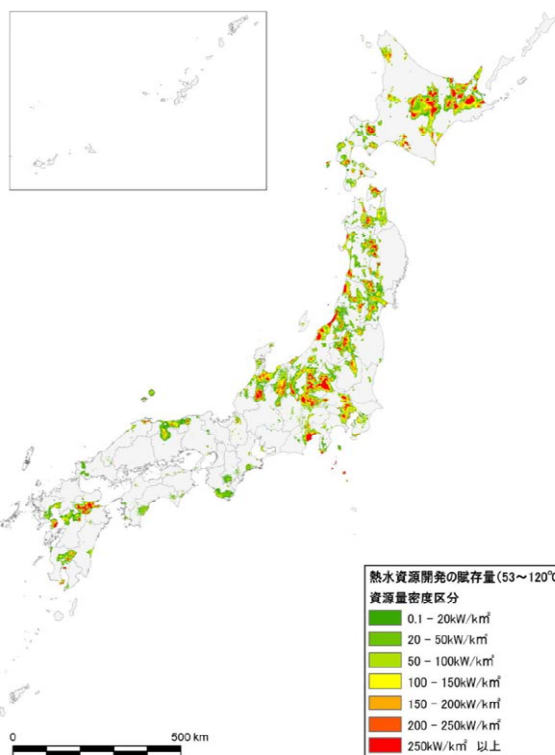
53 ~ 120 の地熱資源
