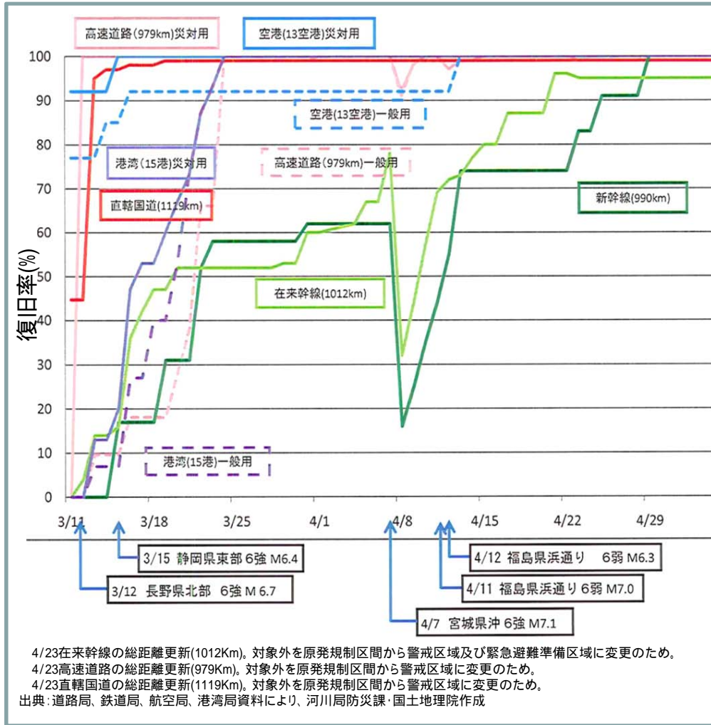
図 交通関係の復旧状況の推移
