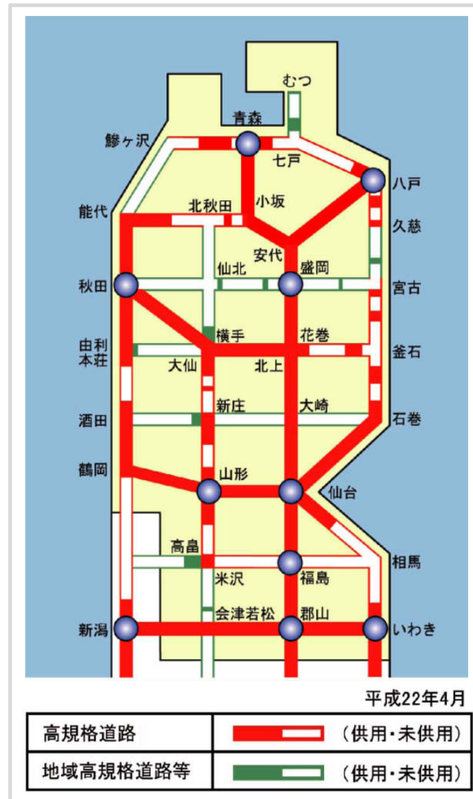
図 東北地方の高規格道路等ネットワーク
